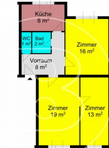
Skizze Grundriss
